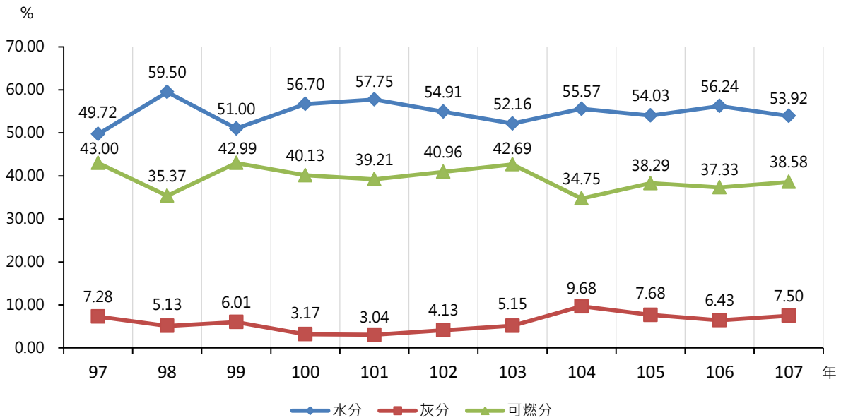
圖二 新北市歷年進廠廢棄物之化學組成比例
