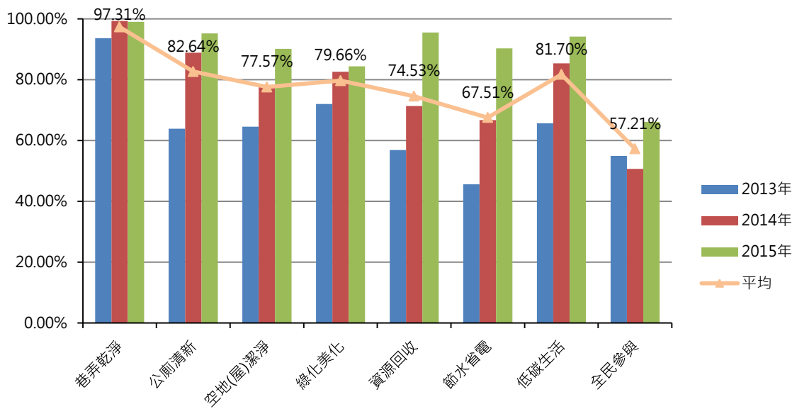
圖一 2013年至2015年各項指標平均通過率
