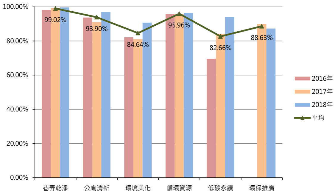
圖二 2016年至2018年各項指標平均通過率
