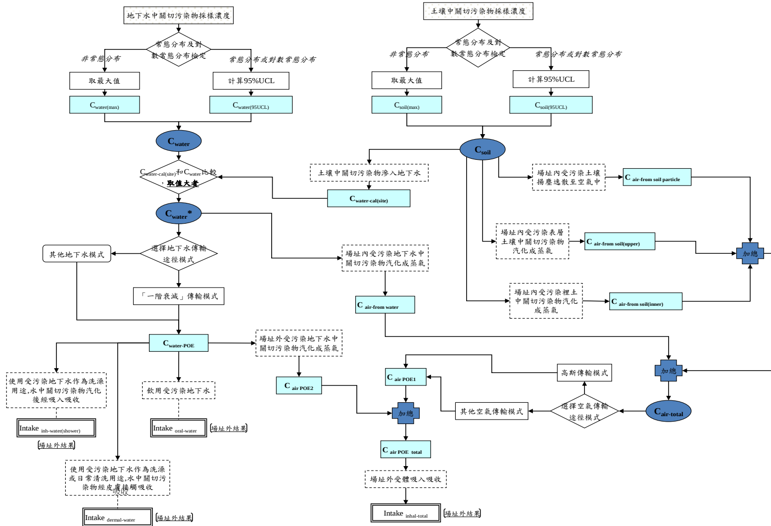
圖3.3.2-2 場址外受體暴露途徑及傳輸途徑評估程序圖
